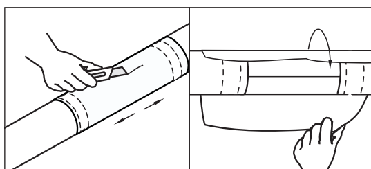
2. Mit einem sehr scharfen Messer die alte Schrumpfmuffe längs durchschneiden. Die Schrumpfmuffe entfernen.
